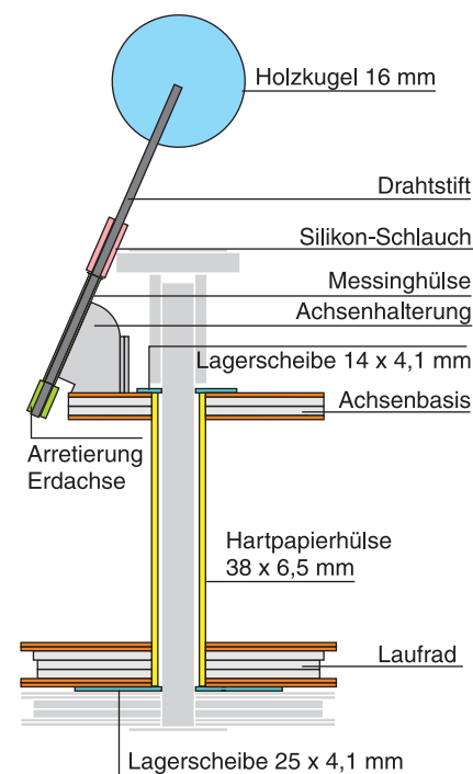
Skizze 7: Erdneigungs-Ausrichtung. (Hell: Erdrotation)
