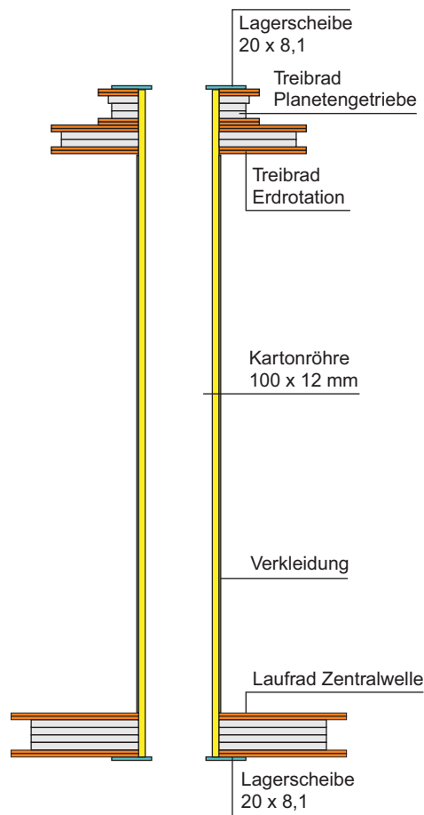
Skizze 4: Zentralwelle
