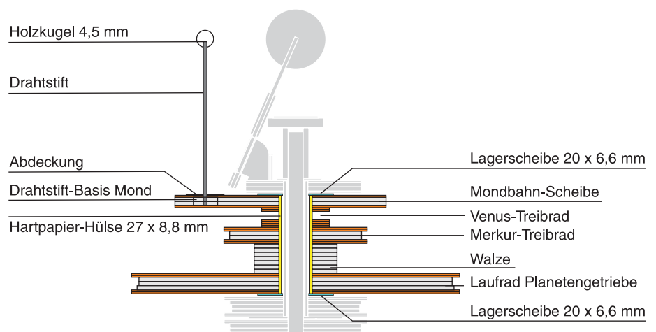
Skizze 6: Planetengetriebe (Hell: Erdneigungs-Ausrichtung und Erdrotation)
